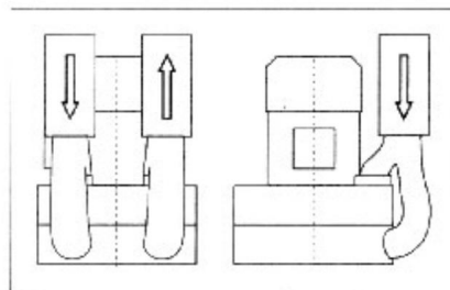
图. 6: 2HB940-BH47(双叶轮大流量规格)
