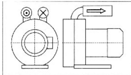
图. 4: 2HB840(双叶轮大流量规格)
