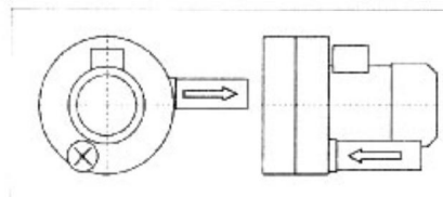
图. 7: 2HB220-2HB920(双叶轮的双段规格)
